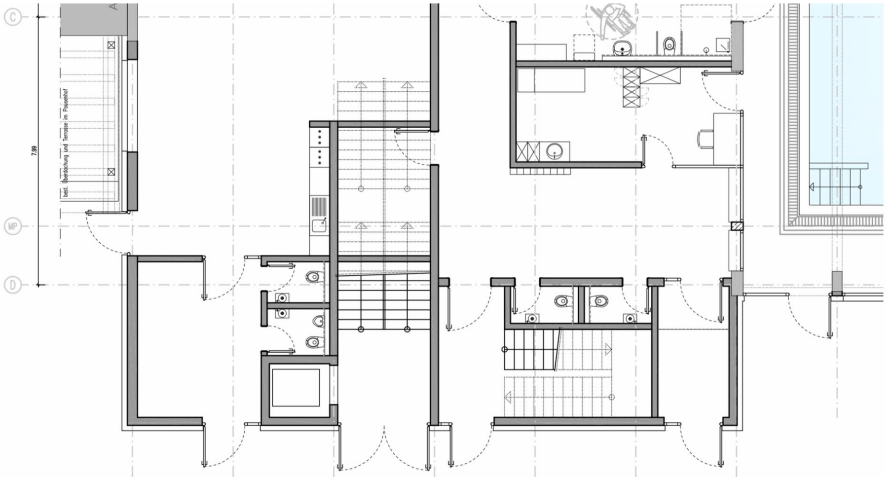
Grundriss Untergeschoss
