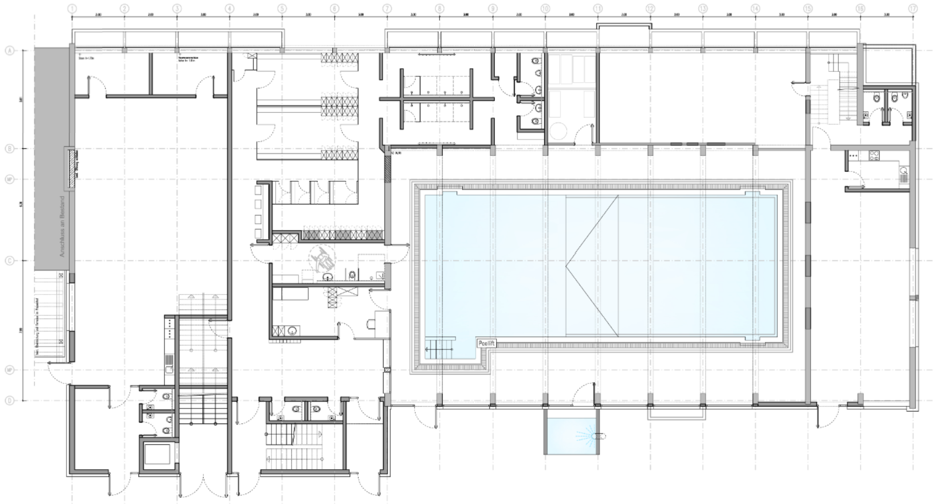
Grundriss Untergeschoss
